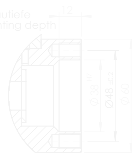
B (1 : 2)
